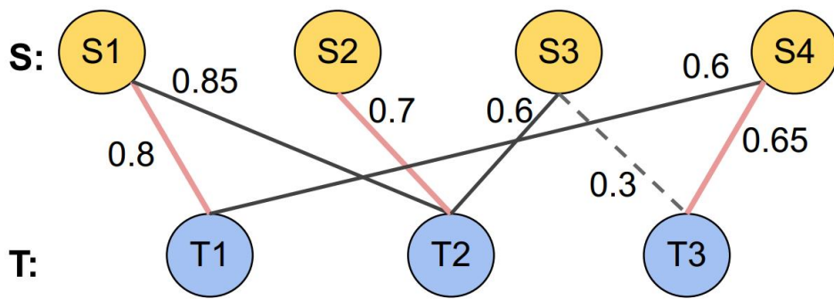
图 3-6 表格相似度得分计算示例
