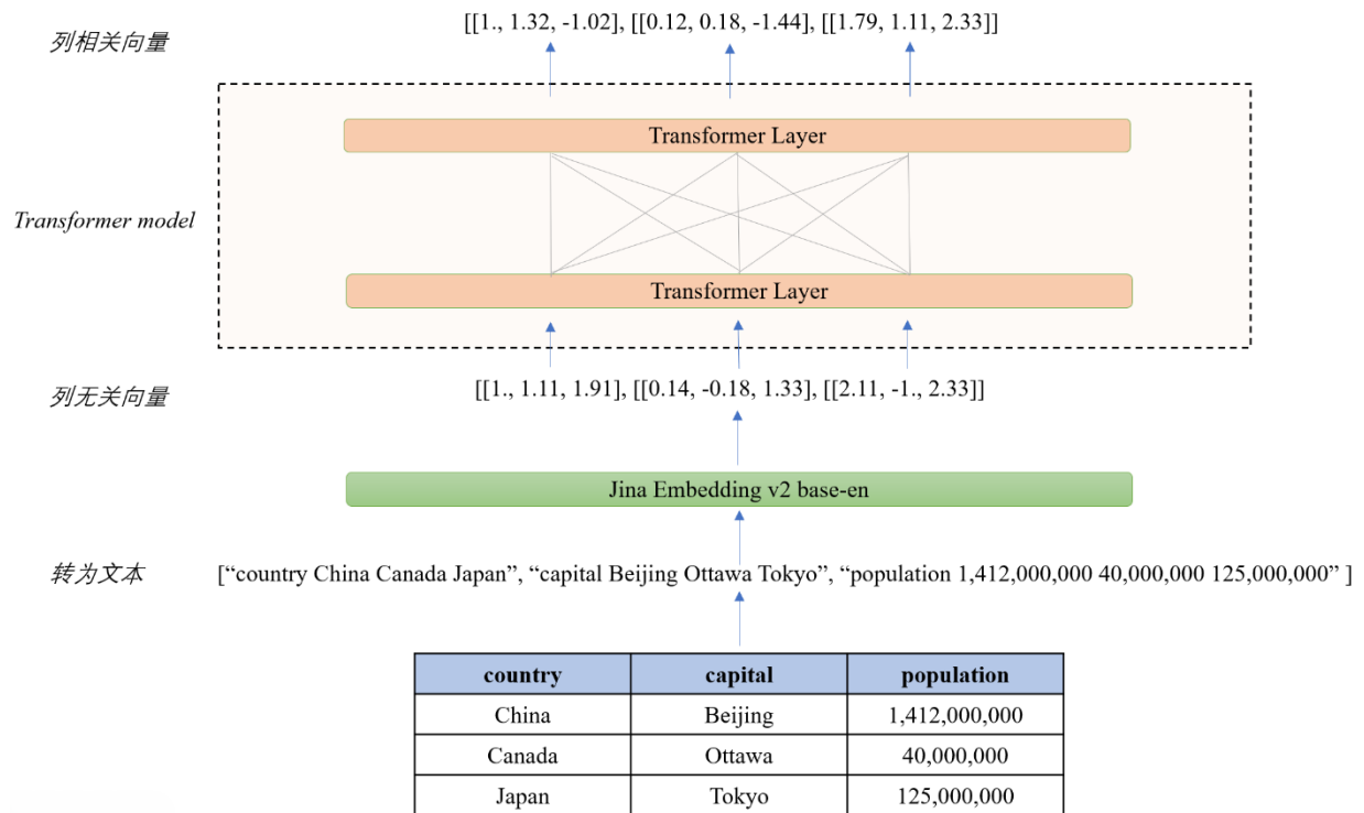
图 3-5 模型架构设计图
