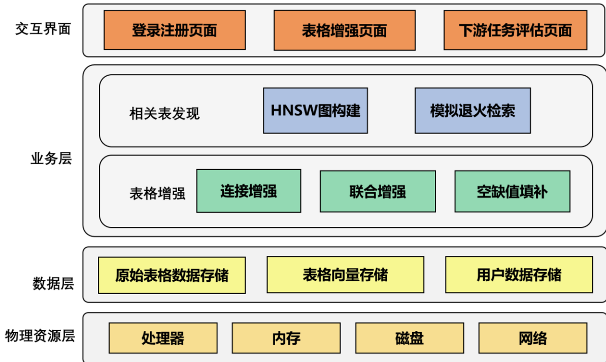
图 3-1 系统架构设计
