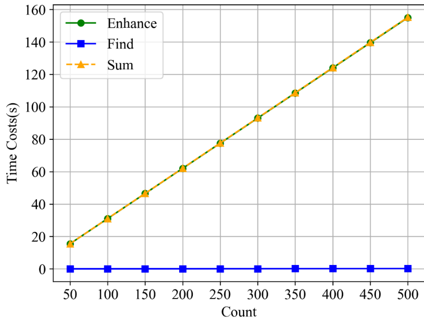
图 4-9 SDASDL 系统在不同表格数量下的耗时曲线
