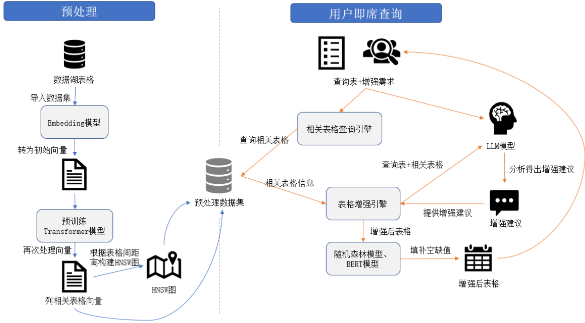
图 3-3 后端系统软件流程图
