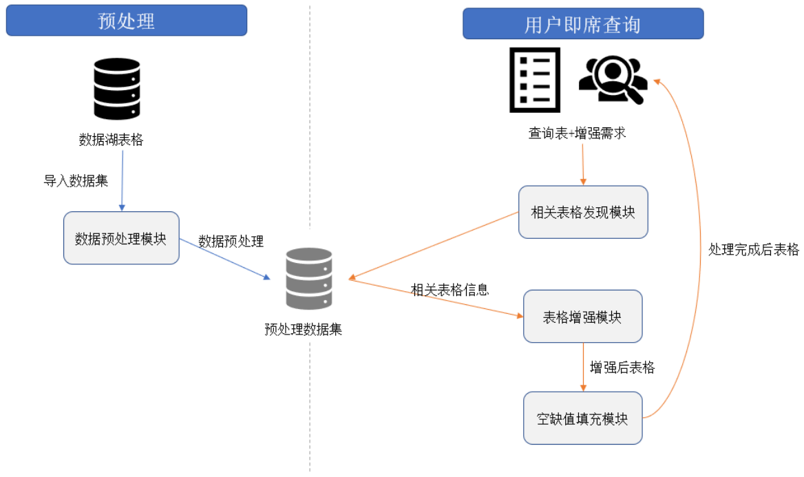
图 3-2 后端系统架构图
