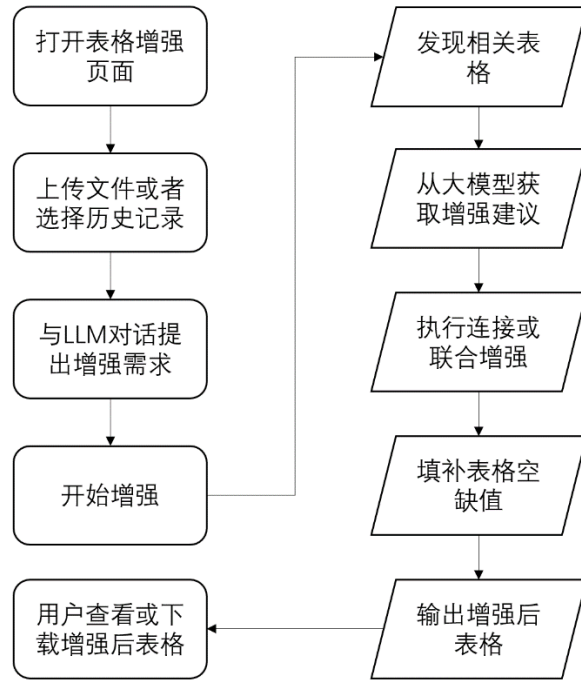
图 4-3 表格增强流程图
