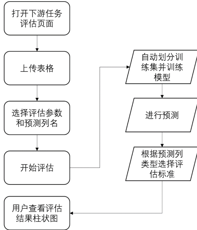
图 4-6 下游任务评估流程图
